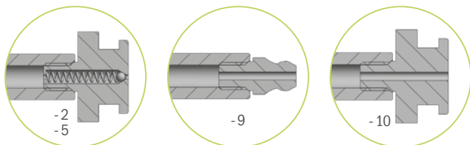
HD-Flachkopfnippel mit Dichtkonus HP pan head nipple with sealing cone
